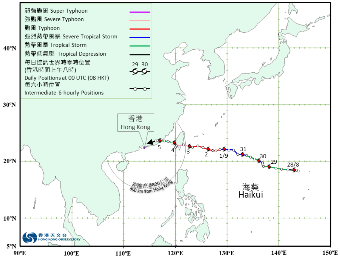
圖 3.4.1a 二零二三年八月二十七日至九月五日海葵(2311)的路徑圖。
